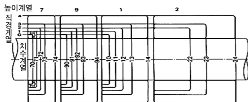
스러스트 베어링의 단면 치수 계열에 의한 구조(단면 계열 5 제외)
