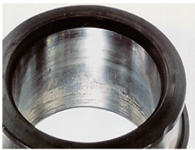
내륜 크립 사례
