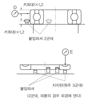
그림 8.1 회전정도의 측정방법(개략)
