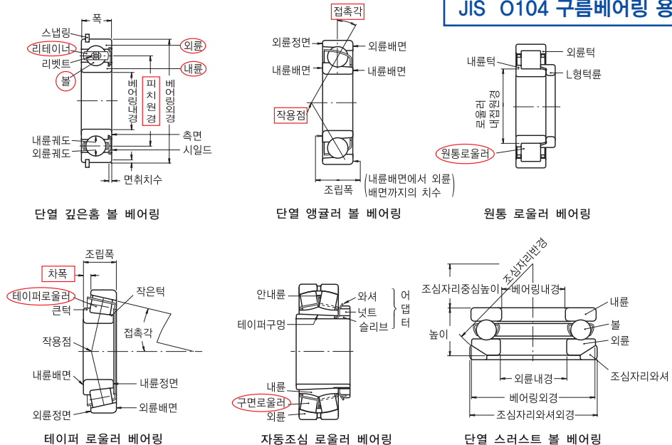
그림 1.1 베어링 각부의 명칭
