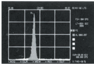
AE를 사용해 미소CRACK의 단계에서 시험을 정지
