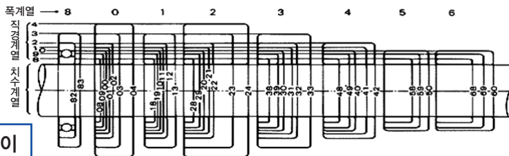
레이디얼 베어링의 단면 치수 계열에 의한 구조(테이퍼 베어링 제외)
