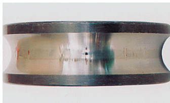
내륜에 발생한 펄스 브리넬링
