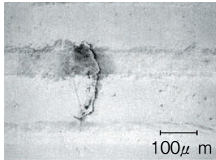
AE를 사용해 미소CRACK의 단계에서 시험을 정지
